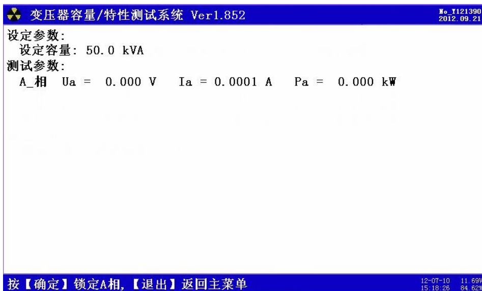
图 13、单相空载—A 相测量
