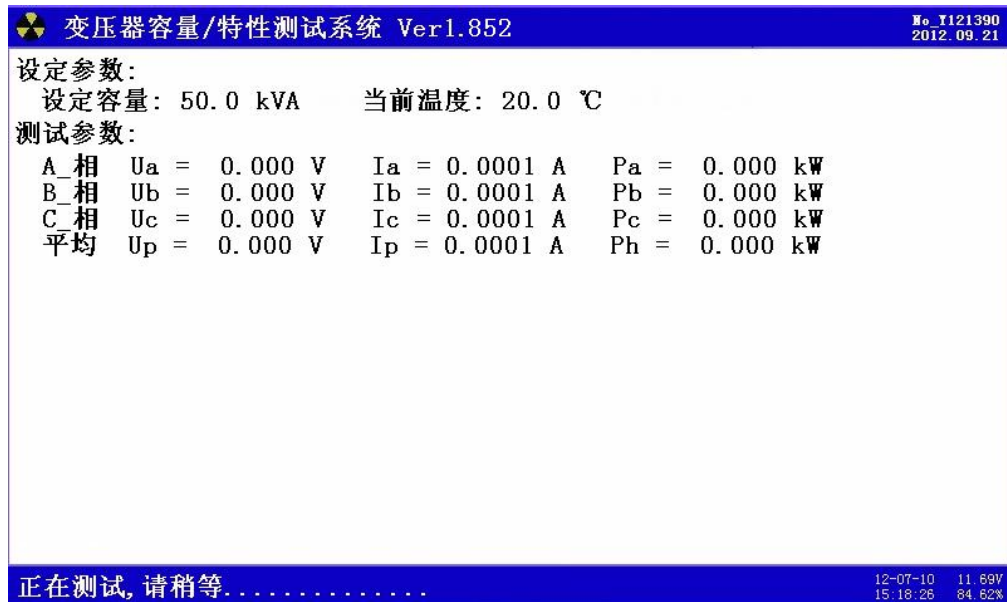
图 10、有源负载测试（进行中）
