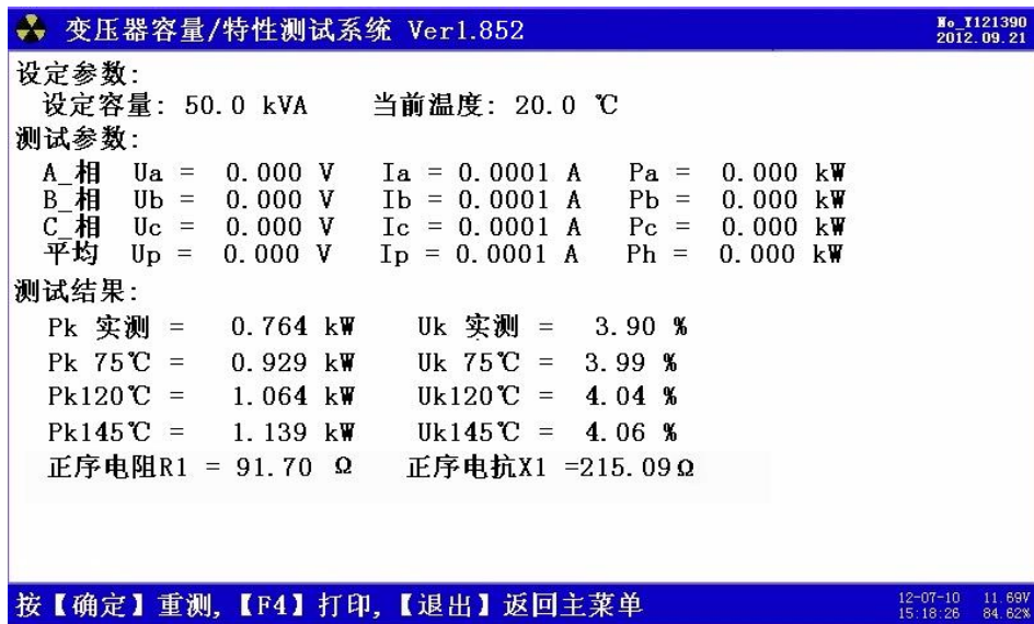
图 12、有源负载测试结果
